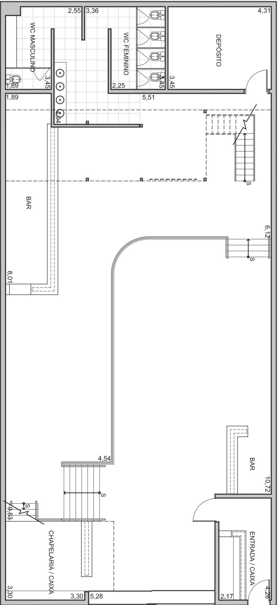
PLANTA BAIXA GERAL ESCALA 1:100
